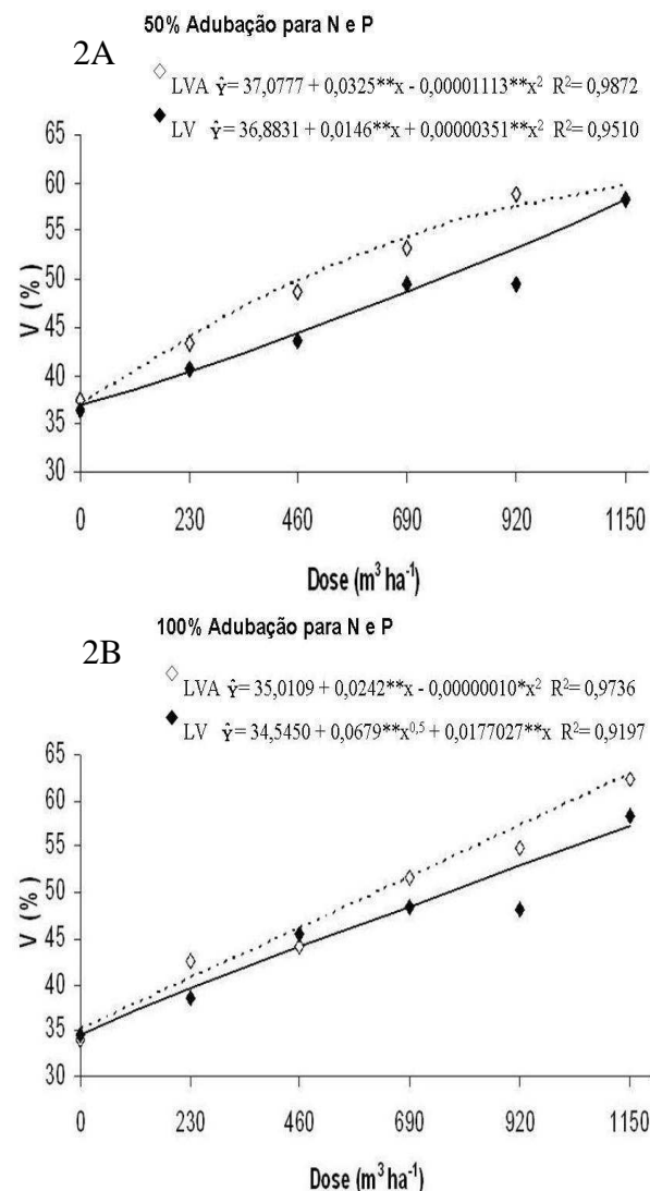
FIGURA 2: Valores de saturação por bases (V) em Latossolo Vermelho-Amarelo (LVA) e Latossolo Vermelho (LV), em função da aplicação de doses de vinhaça e dos níveis de adubação química, 50% (Figura 2A) e 100% (Figura 2B), após o cultivo de Brachiaria brizantha . * e ** significativo à 5 e à 1% de probabilidade pelo teste t, respectivamente.
