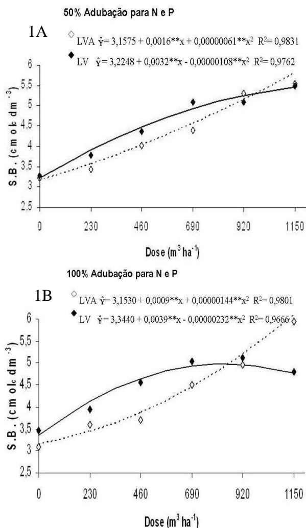
FIGURA 1: Valores de soma de bases (S.B.) em Latossolo Vermelho-Amarelo (LVA) e Latossolo Vermelho (LV), em função da aplicação de doses de vinhaça e dos níveis de adubação química, 50% (Figura 1A) e 100% (Figura 1B), após o cultivo de Brachiaria brizantha . ** significativo a 1% de probabilidade pelo teste t.
