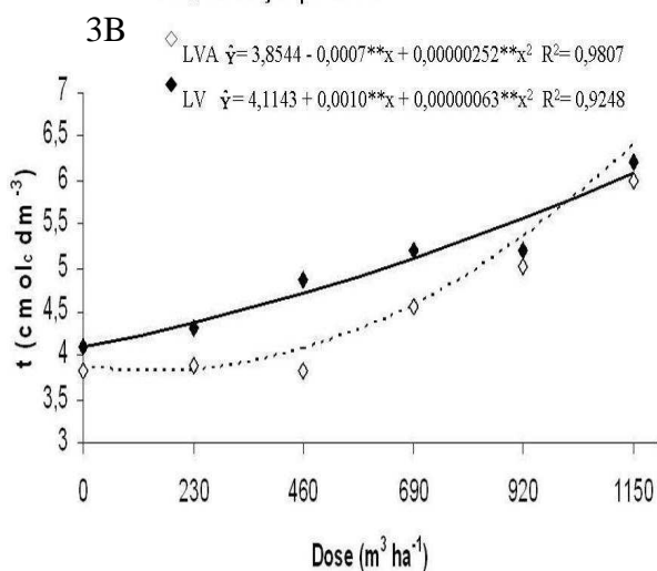
FIGURA 3: Valores de capacidade de troca catiônica efetiva (t), em Latossolo Vermelho-Amarelo (LVA) e Latossolo Vermelho (LV), em função da aplicação de doses de vinhaça e dos níveis de adubação química, 50% (Figura 3A) e 100% (Figura 3B), após o cultivo de Brachiaria brizantha . ** significativo a 1% de probabilidade pelo teste t.
