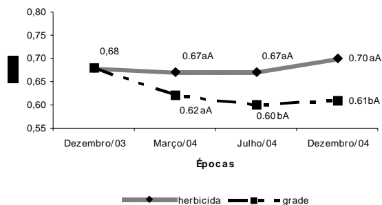
Figura 4 – Diâmetro médio geométrico (DMG) na região rodado do trator, na camada 20 a 40 cm. Letra minúscula comparam os sistemas de manejo grade e herbicida e maiúscula a época dentro de cada sistema. Valores seguidos de mesma letra não diferem entre si, pelo teste t- Student, a 5%, CV= 16%
