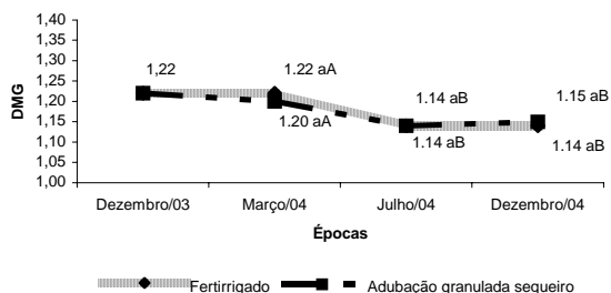
Figura 5 – Diâmetro médio geométrico (DMG) na região sob copa do cafeeiro, na camada 0 a 20 cm. Letra minúscula comparam os sistemas de manejo fertirrigado e adubação granulada de sequeiro e maiúscula a época dentro de cada sistema. Valores seguidos de mesma letra não diferem entre si, pelo teste t- Student a 5%, CV= 10%.
